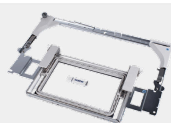
VRBF180 180 x 100mm Båndramme
